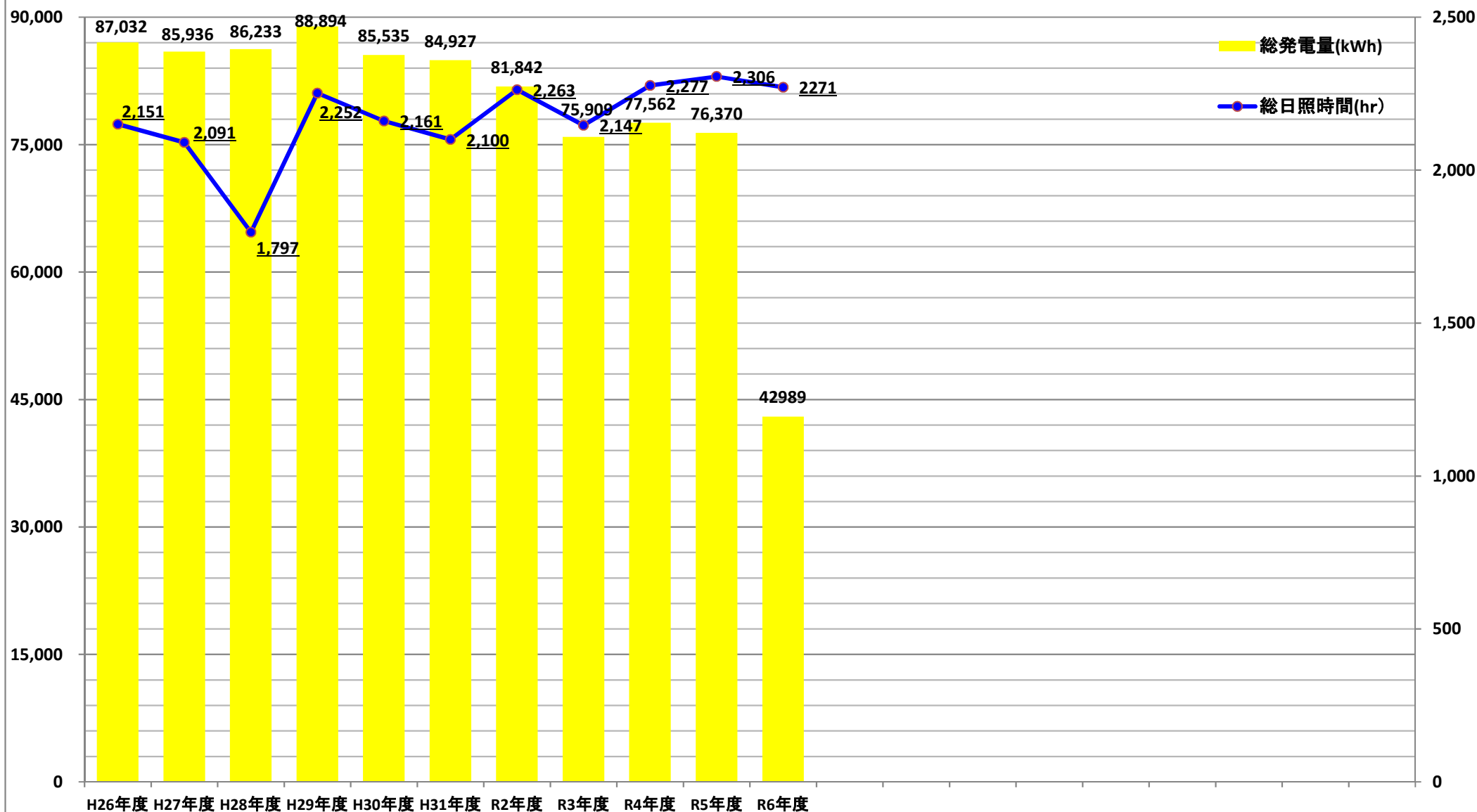
尼崎市立クリーンセンター太陽光発電所の総日照時間と総発電量の関係
