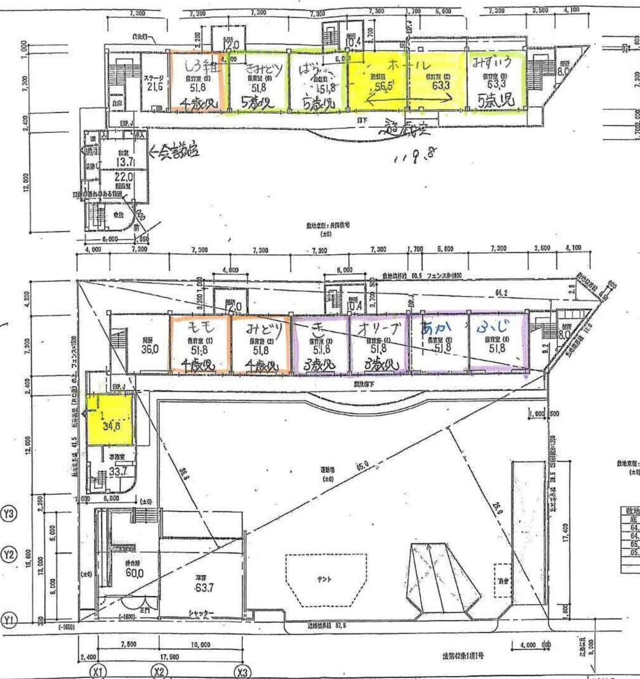
配置図
