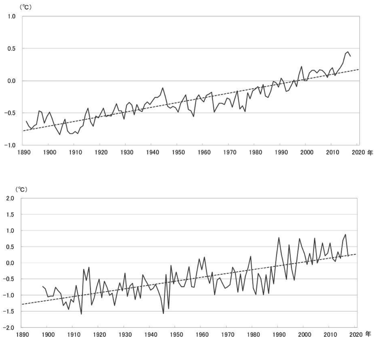
図1-4 平均気温偏差の推移（上：世界、下：日本）
