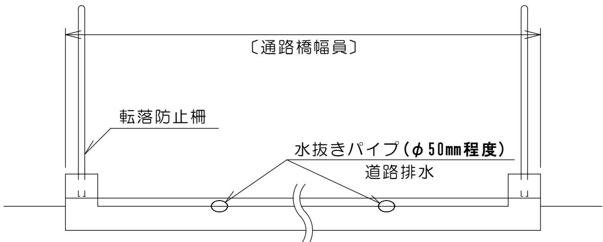
正面図
