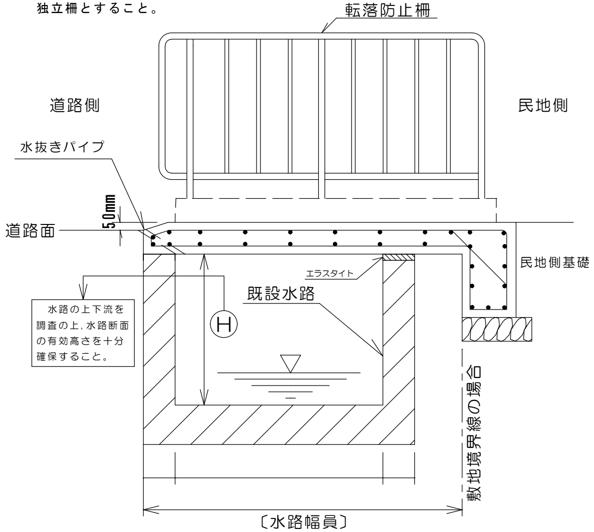
断面図
