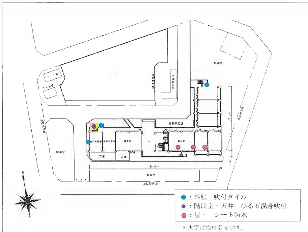
図 4-1 (21) 試料採取地点 (西川平七改良住宅)
