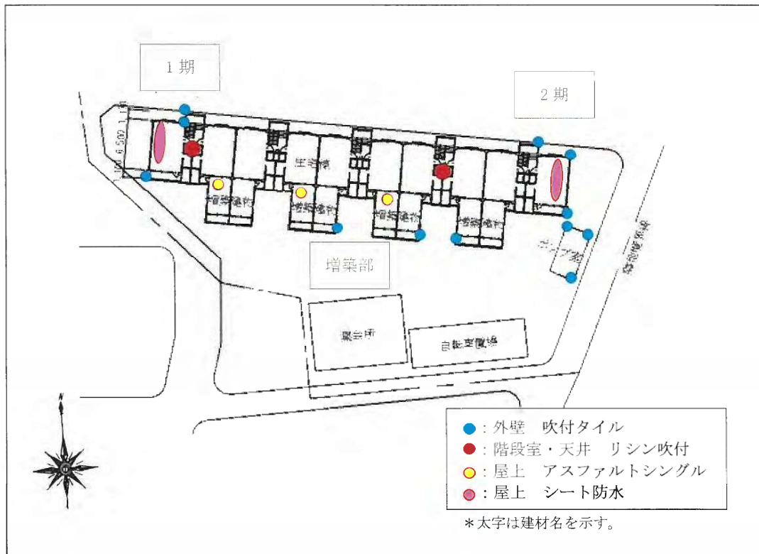
図 4-1 (19) 試料採取地点 (西川住宅)
