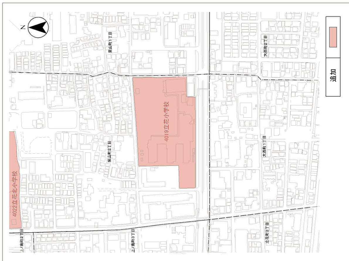
計画図(案) S=1:2,500 4019号 立花小学校
