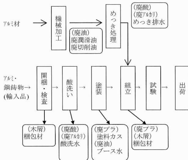
図4. 電力用開閉装置製造フローシート(铸件品の場合)
