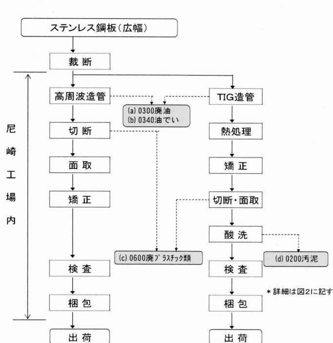
図1 ステンレス鋼管製造フロー
