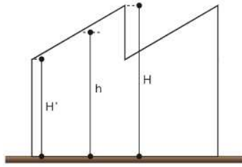
(その3) のこぎり形天井等の例
