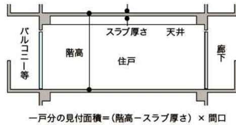
（断面図）
